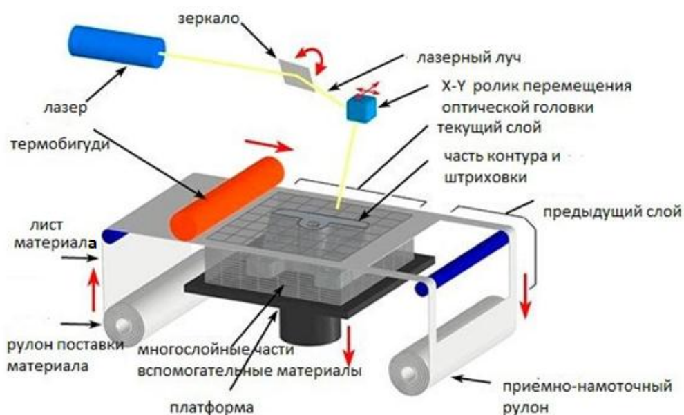
Рис. 2.24. Схема процесса ламинирования
