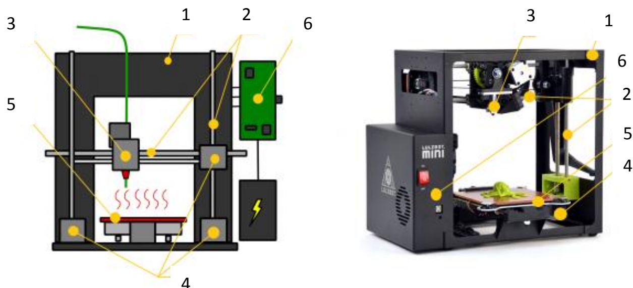
Рис. 2.1. Схема устройства 3D-принтера экструзивного типа: 1 – корпус, 2 – закрепленные на нем направляющие, 3 – печатающая головка, 4 – шаговые двигатели, 5 – рабочий стол; 6 – управляющая электроника
